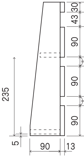
側面図
